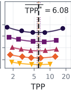
Untied-2
