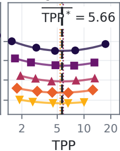
Deep Vanilla
