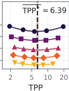
Loop-2
