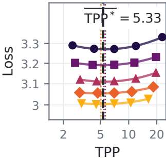
Vanilla
