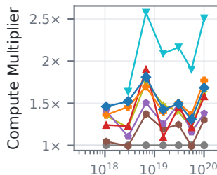
CORE NLL
