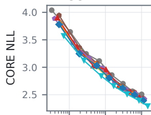
CORE NLL
