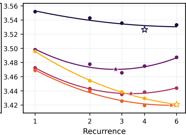
Untied-2 optima
