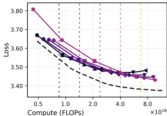
Tied Vanilla optima
