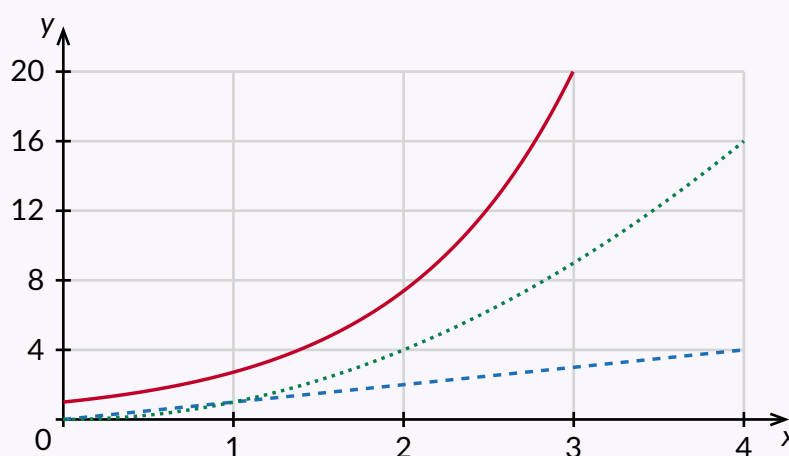
e^x (rouge), x (bleu pointillé), x^2 (vert).
