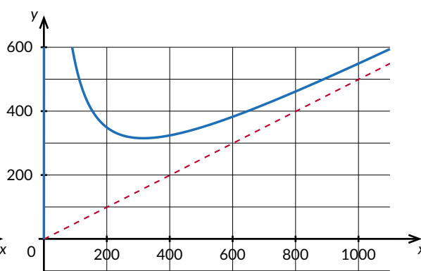
graphique de g
