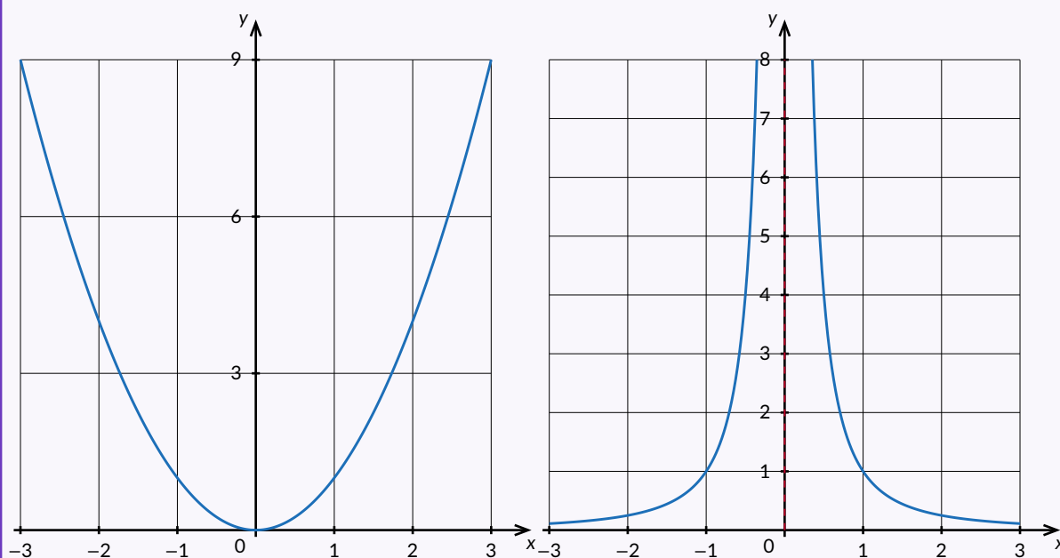
fonction de référence x^2
