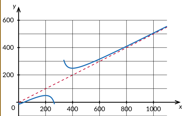
graphique de f
