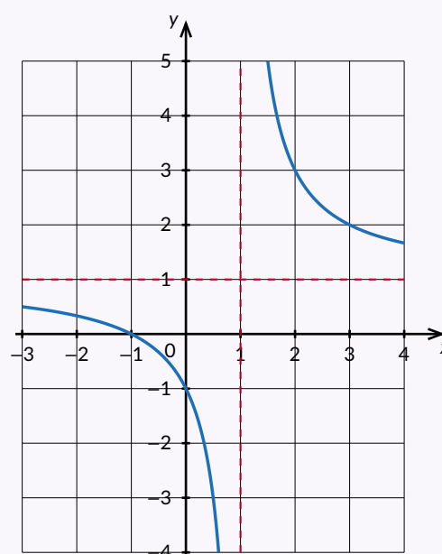
k(x) = \frac{x+1}{x-1} : une A.V.
