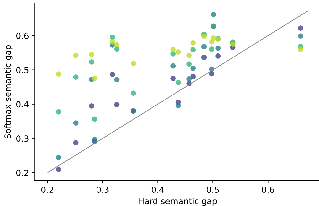
raw softmax
