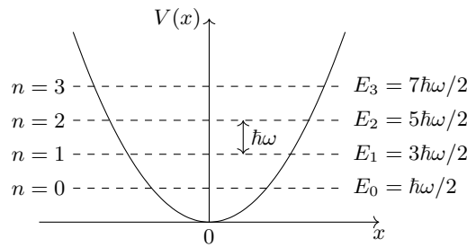
FIGURE 5 – Potentiel harmonique.
