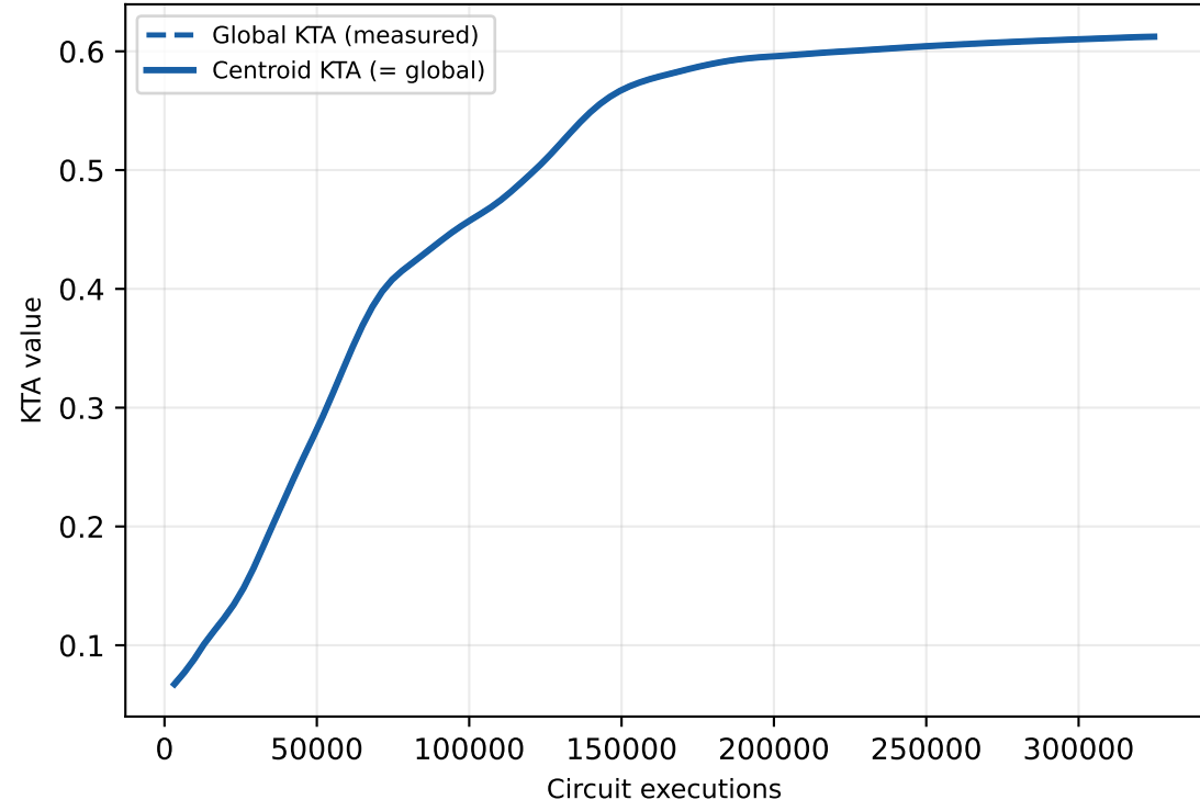
CCKA (ours)
