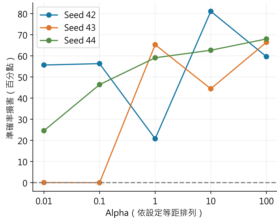
實驗 A：各 seed 的結果
