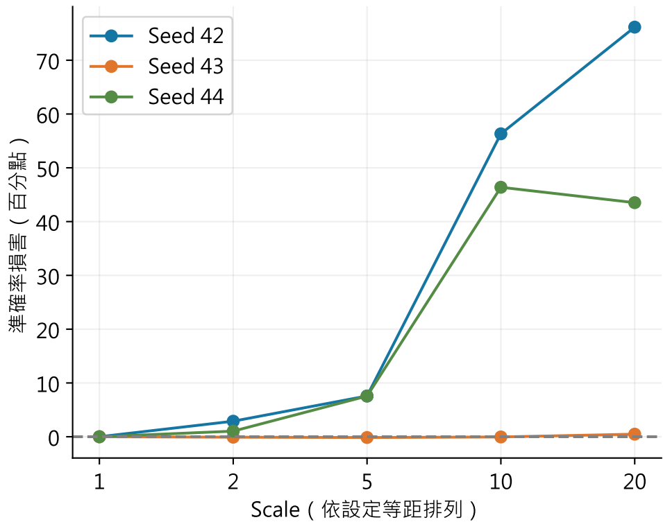
實驗 B：各 seed 的結果
