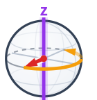
zじくのまわりを半周
