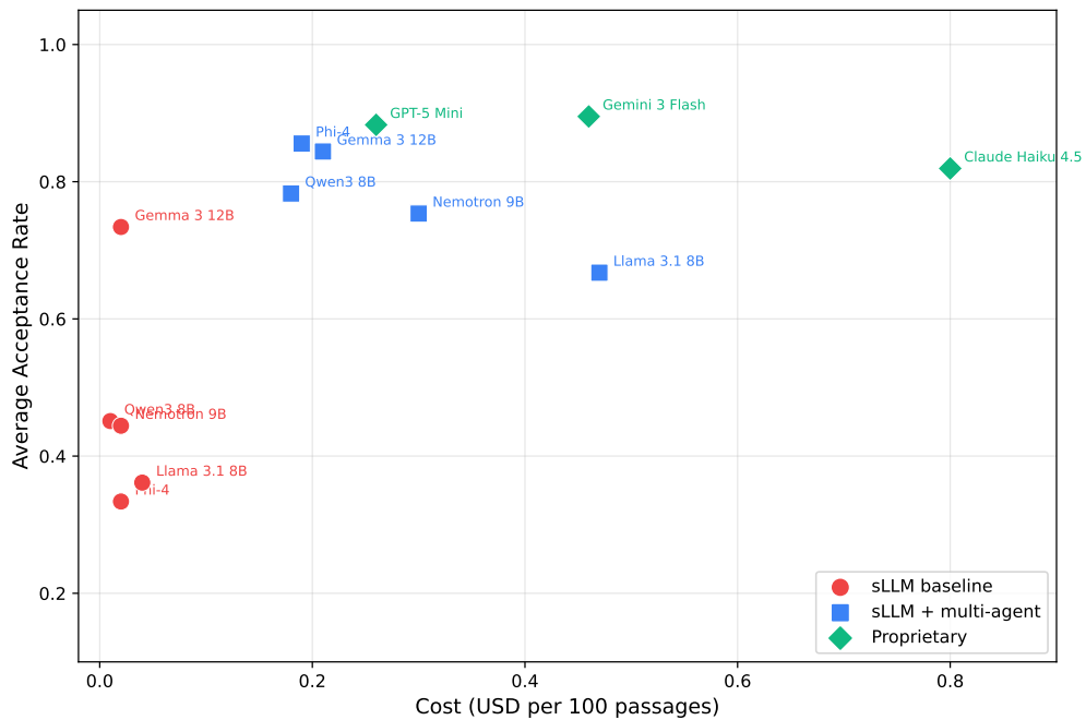
Hình 5.3: Biểu đồ phân tán chi phí API (USD) so với Acceptance trung bình trên ba cấp độ nhận thức, xác định biên Pareto tối ưu giữa chất lượng và ngân sách
