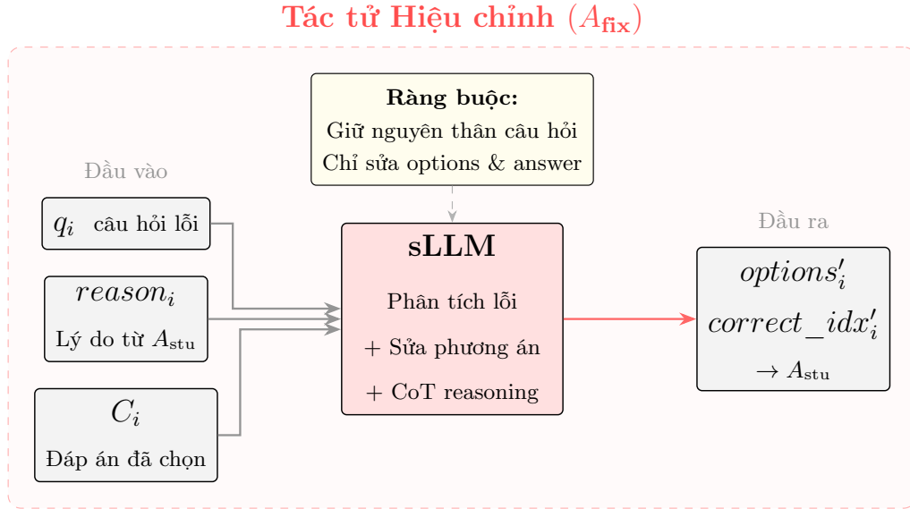
Hình 3.5: Luồng xử lý bên trong Tác tử Hiệu chỉnh: nhận câu hỏi lỗi kèm lý do từ Tác tử Học sinh, chỉ sửa phương án và đáp án, đưa lại để tái kiểm định
