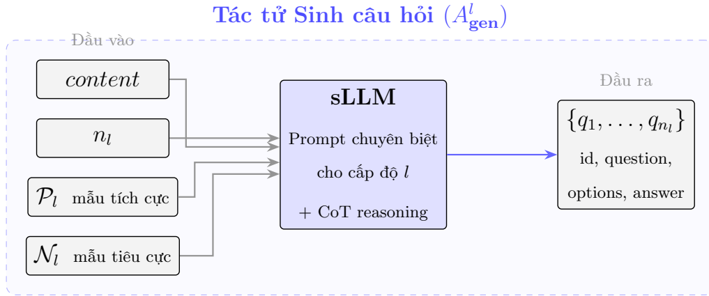
Hình 3.2: Luồng xử lý bên trong Tác tử Sinh câu hỏi: nhận văn bản nguồn và mẫu tham chiếu, sinh câu hỏi qua sLLM với prompt chuyên biệt theo cấp độ
