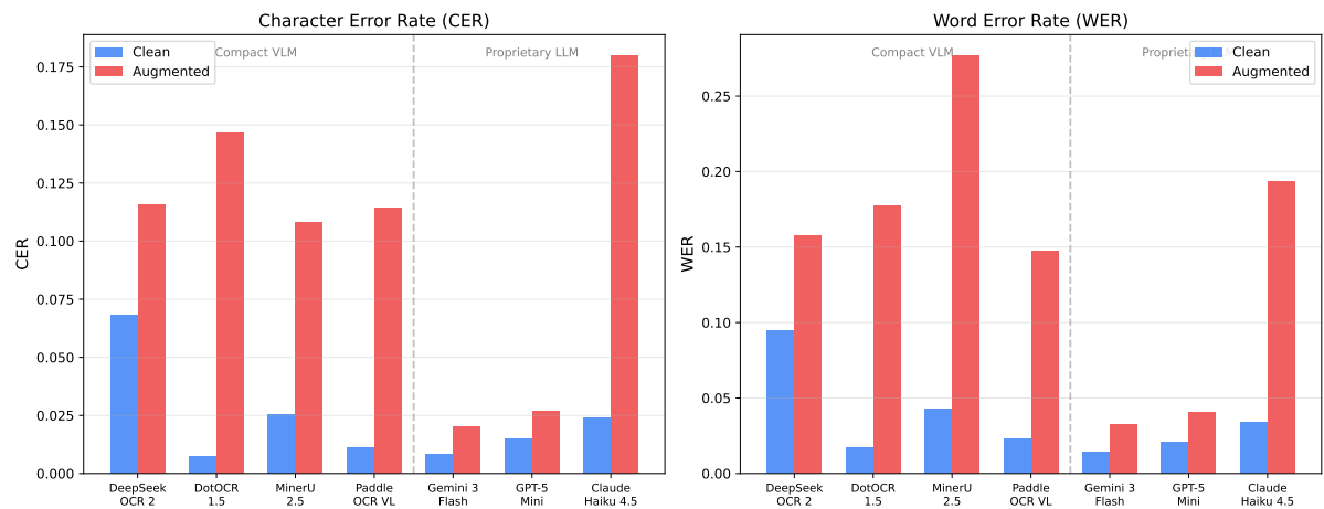
Hình 5.2: So sánh CER và WER giữa điều kiện ảnh sạch và ảnh nhiễu cho bảy mô hình OCR, minh họa mức độ suy giảm hiệu suất khi chuyển sang điều kiện thực tế
