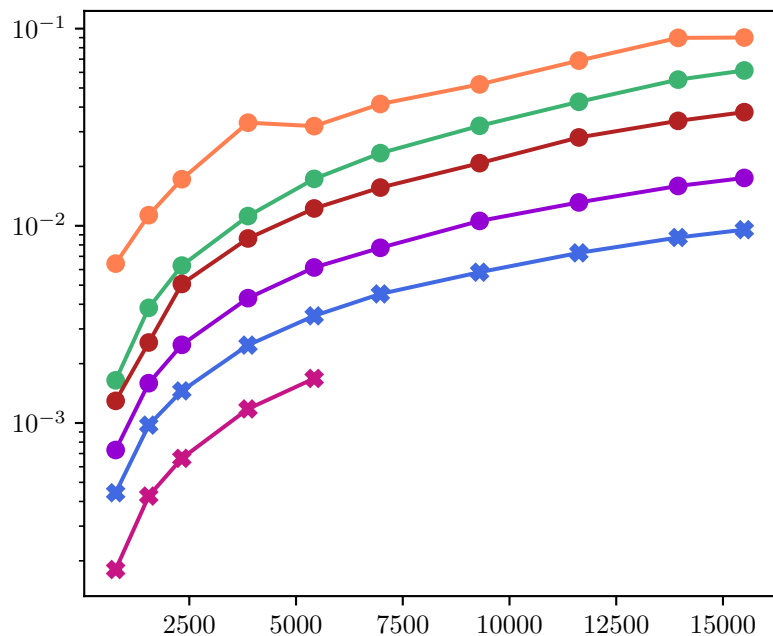
Group Lasso
