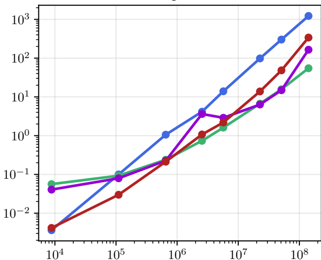
Group Lasso
