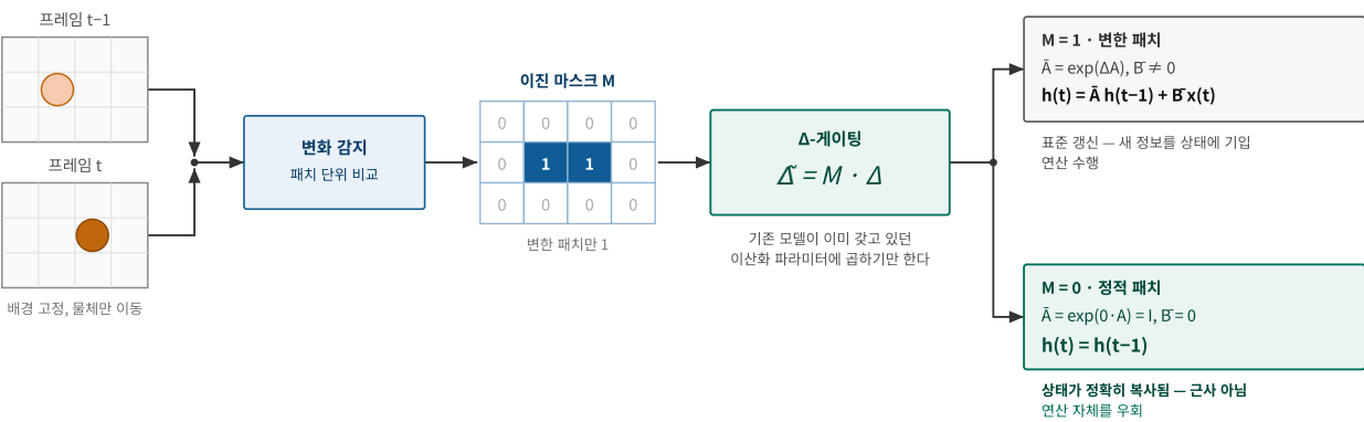
Figure. Δ-게이팅 — 마스크를 이산화 파라미터에 곱하면 연산 스킵이 곧 상태 보존이 된다
