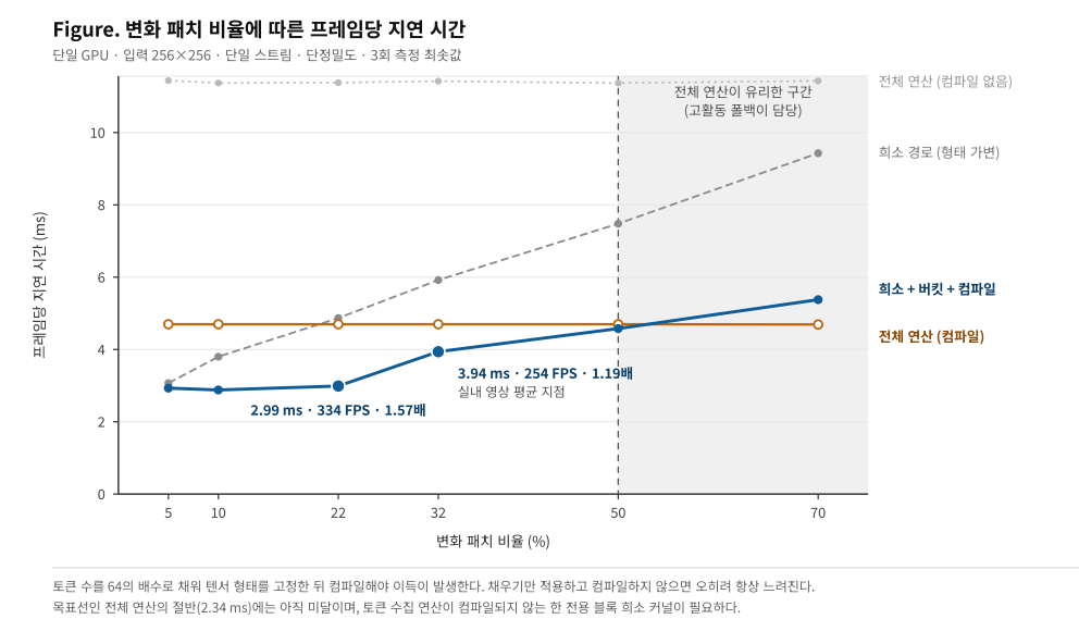
그림 4. 변화 패치 비율에 따른 프레임당 지연 시간 — 세로 점선이 회소 경로와 전체 연산의 성능이 같아지는 지점.
