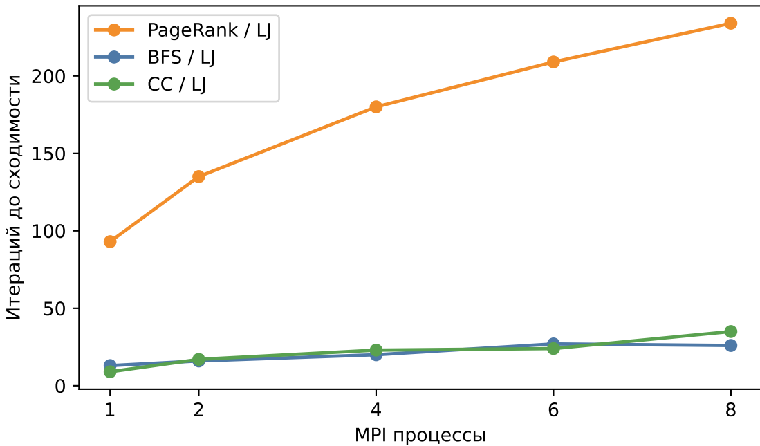
Число итераций vs. число MPI-процессов (граф LiveJournal)
