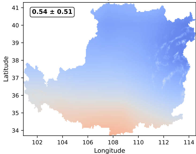
SSP5-8.5 April-October
