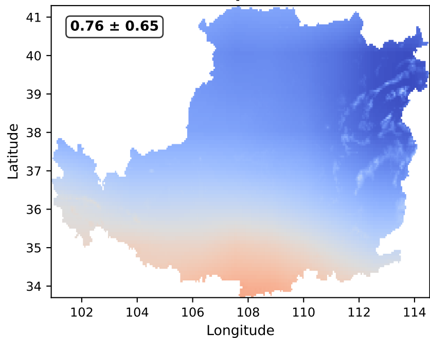
SSP5-8.5 April-October
