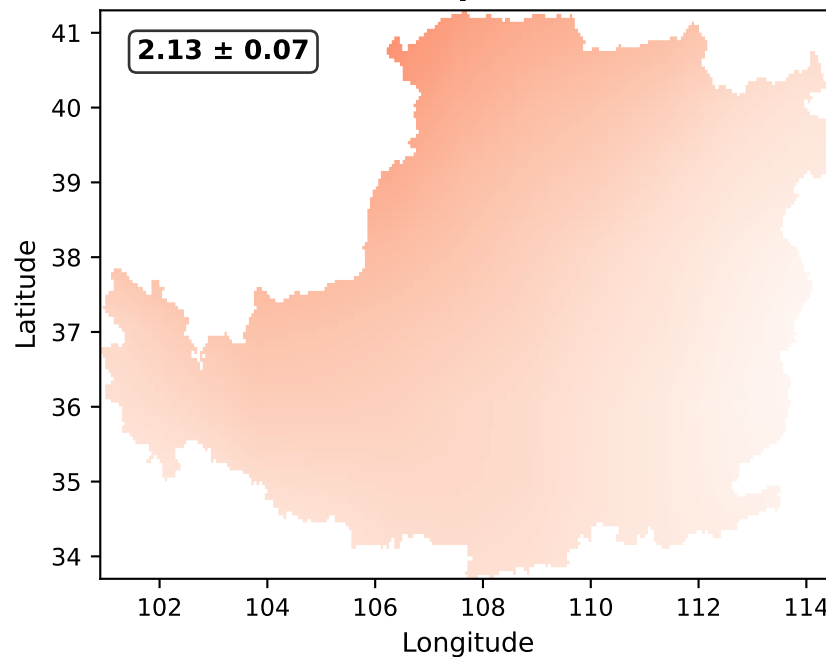
SSP5-8.5 April-October
