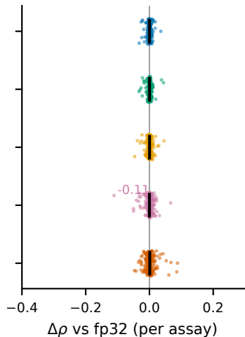
ESM2-15B
