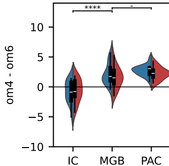
C aPE
