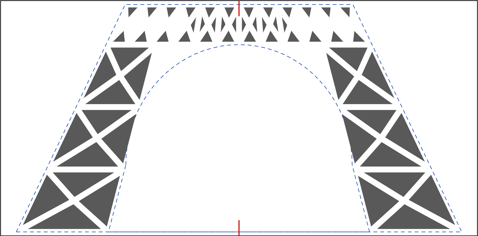
POCHOIR T1 · sert pour les 4 faces du tronçon 1
