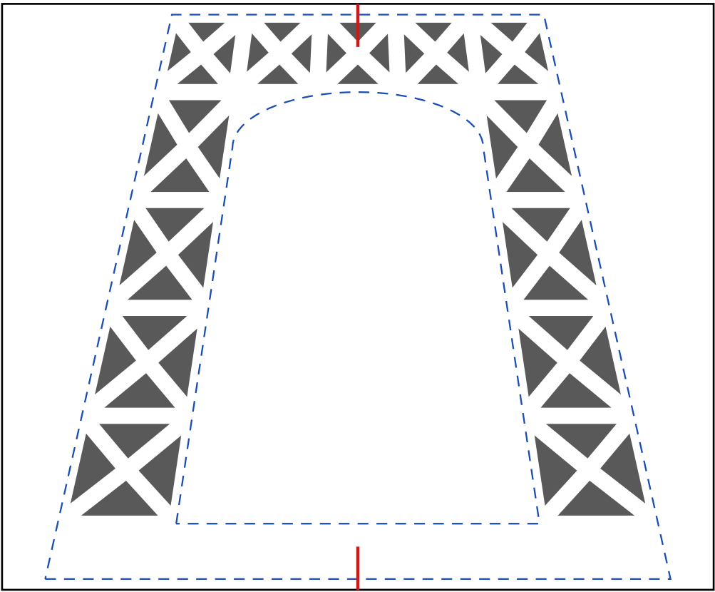
POCHOIR T2 · sert pour les 4 faces du tronçon 2
