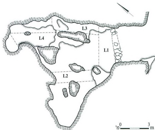
תוכנית 7. מערה 46/VI.
