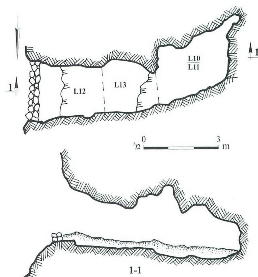
תוכנית 3. מערה 7/IV: תוכנית ותחת.
