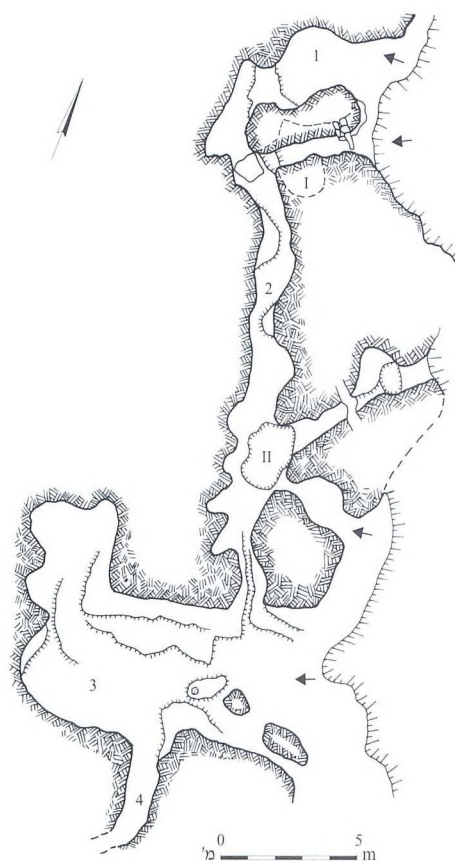
תוכנית 8. מערה 52/VI.
