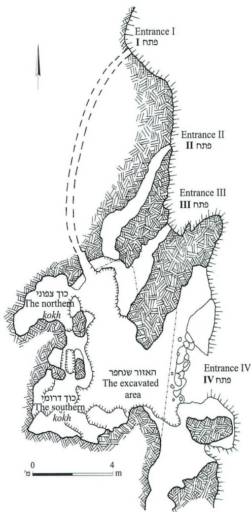
תוכנית 6. מערה 43/VI.
