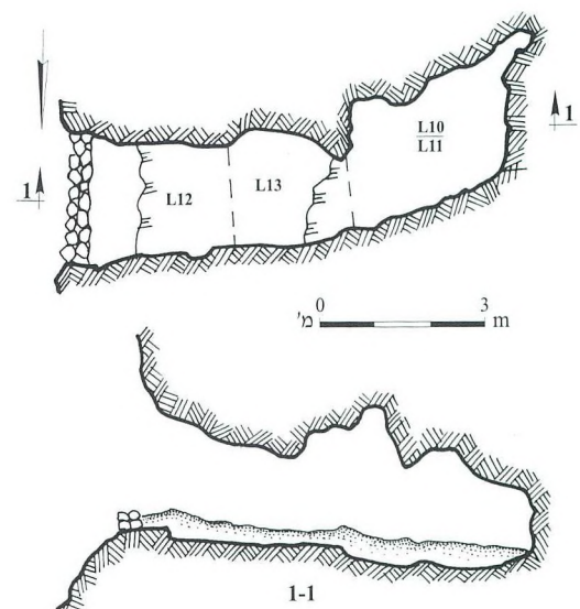
תוכנית 3. מערה 7/IV: תוכנית ותחת.
