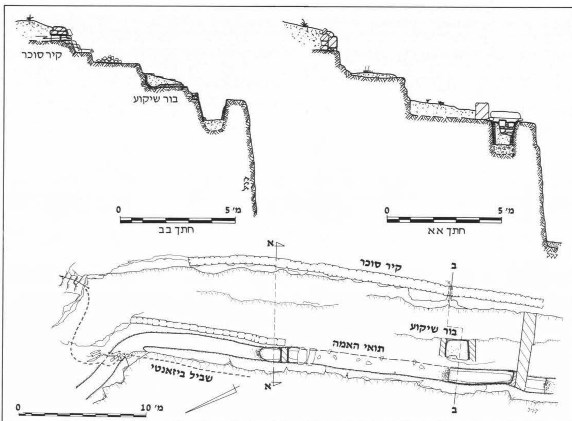
איור 5: האמה הדרומית, תכנית וחיתכי רוחב (נק' 11)
