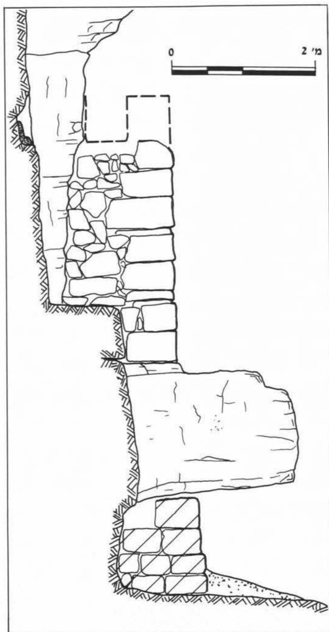
איור 8: האמה הדרומית, חתך (נק' 15)
