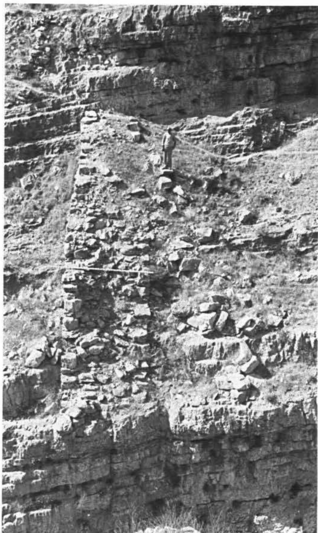
איור 9: יסודות של גשר באמה הדרומית (נק' 34), מבט לצפון
