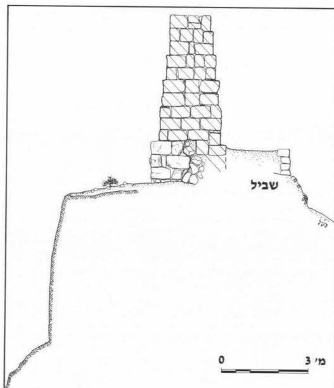
איור 21: הגשר המזרחי, חתך בחלקו המערבי (נק' 48)
