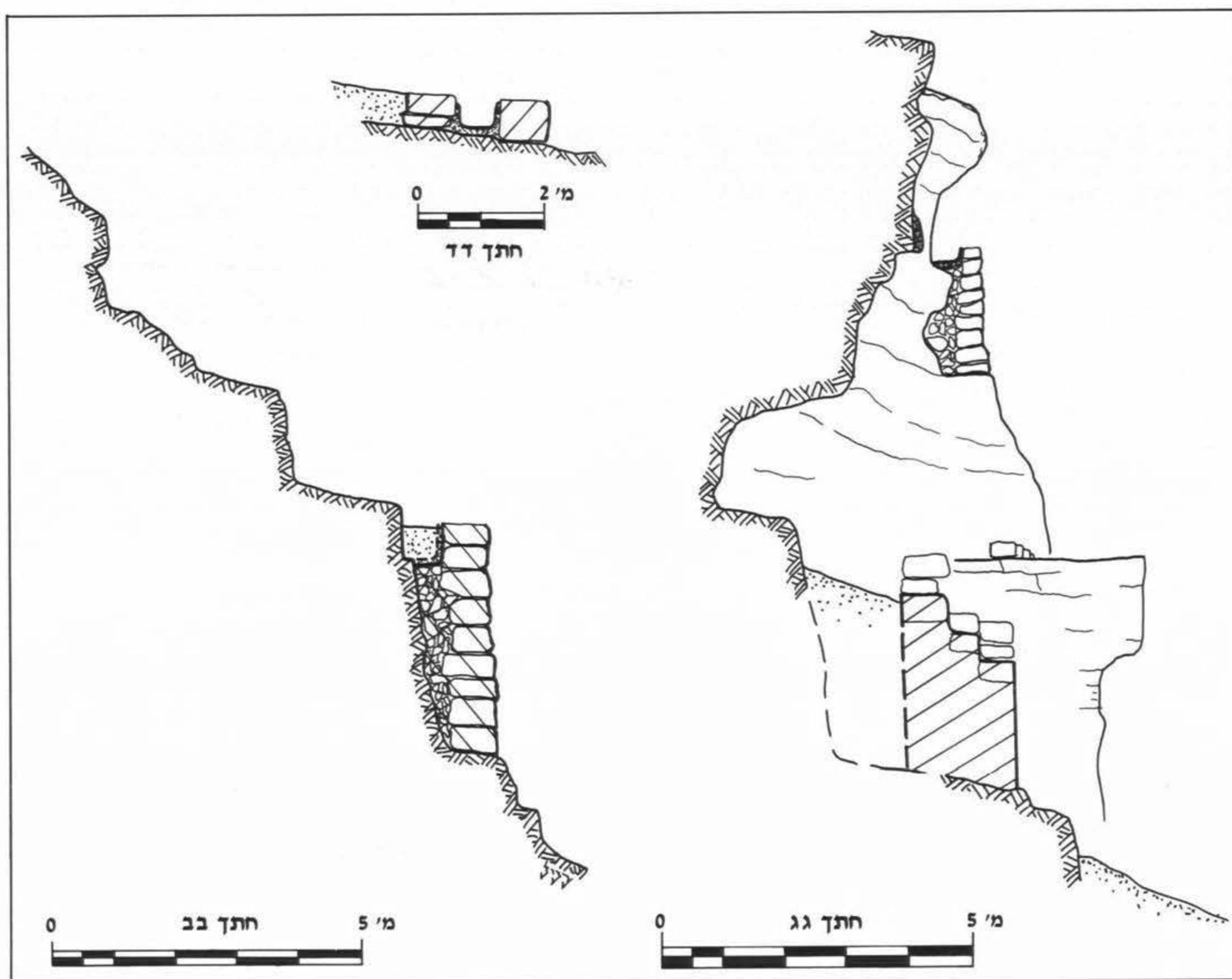
איור 13: האמה הדרומית, חתכים (נק' 40)
