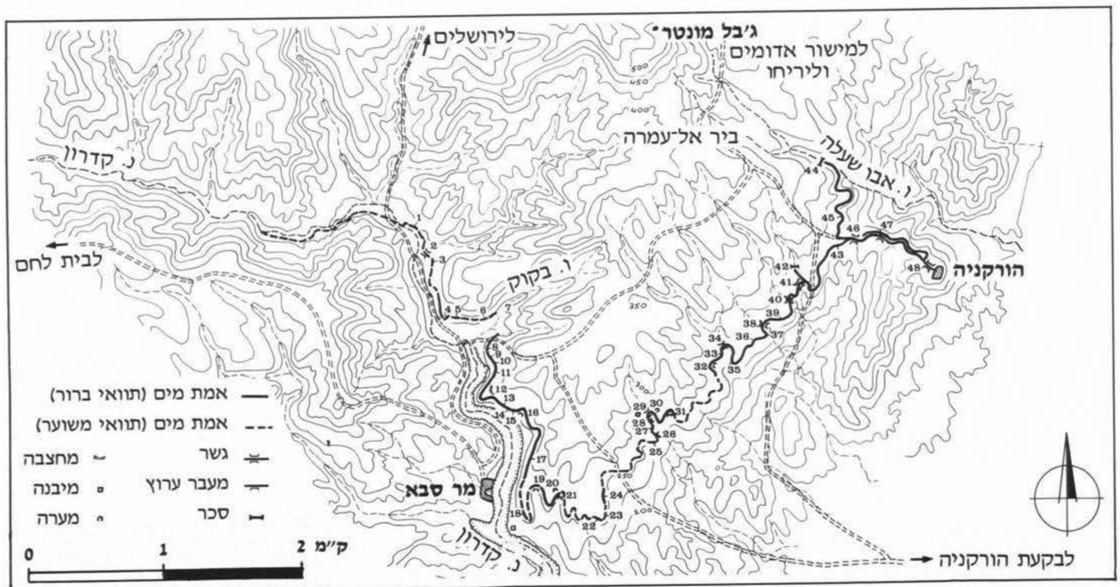
איור 1: מערכת אמות המים של הורקניה
