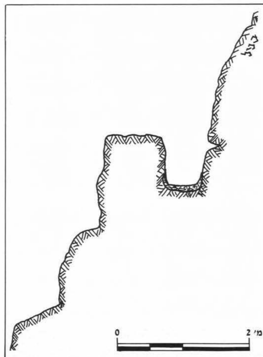
איור 3: האמה הדרומית, חתך (נק' 9)
