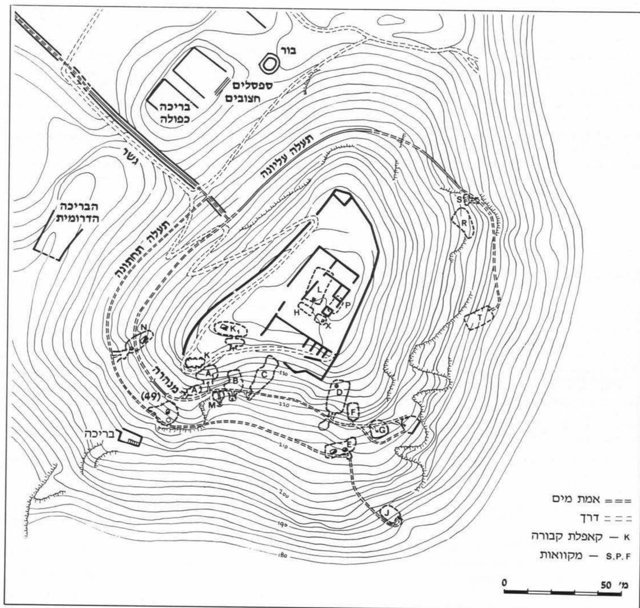
איור 22: מערכת הבורות ובריכות המים של הורקניה
