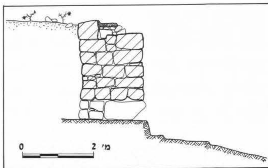
איור 7: האמה הדרומית, חתך (נק' 14)
