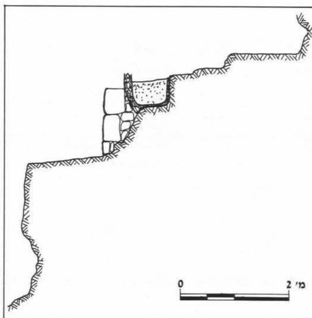
איור 4: האמה הדרומית, חתך (נק' 10)
