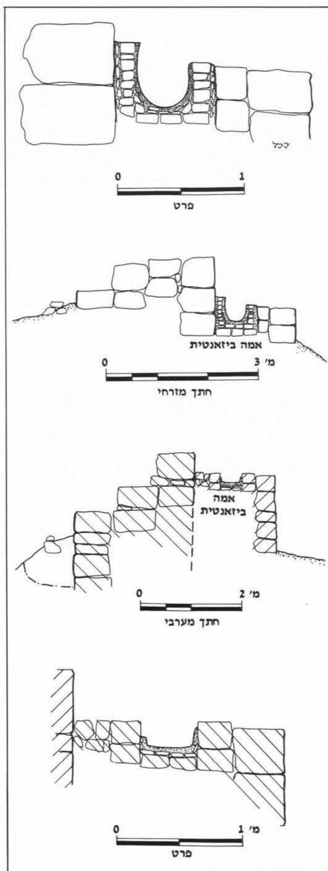
איור 16: האמה הצפונית, חתכים
