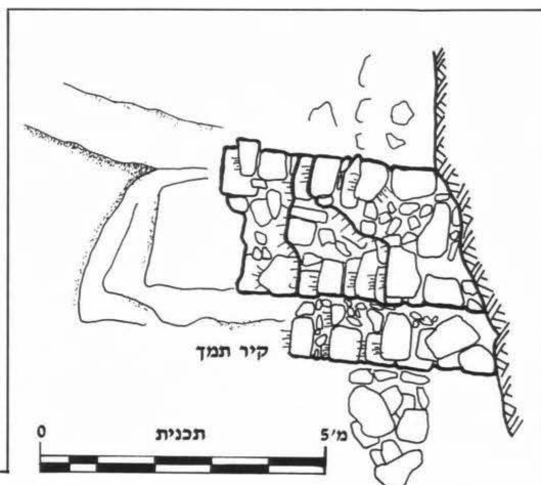
איור 11: האמה הדרומית, תכנית (נק' 40)
