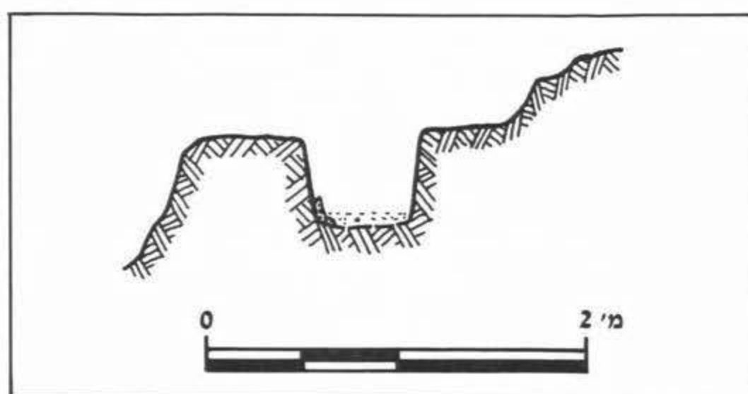
איור 10: האמה הדרומית, חתך (נק' 35)
