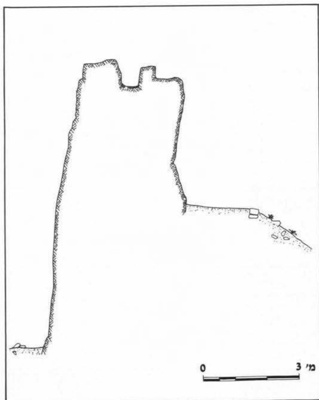
איור 18: הגשר המזרחי, חתך בחלקו המזרחי
