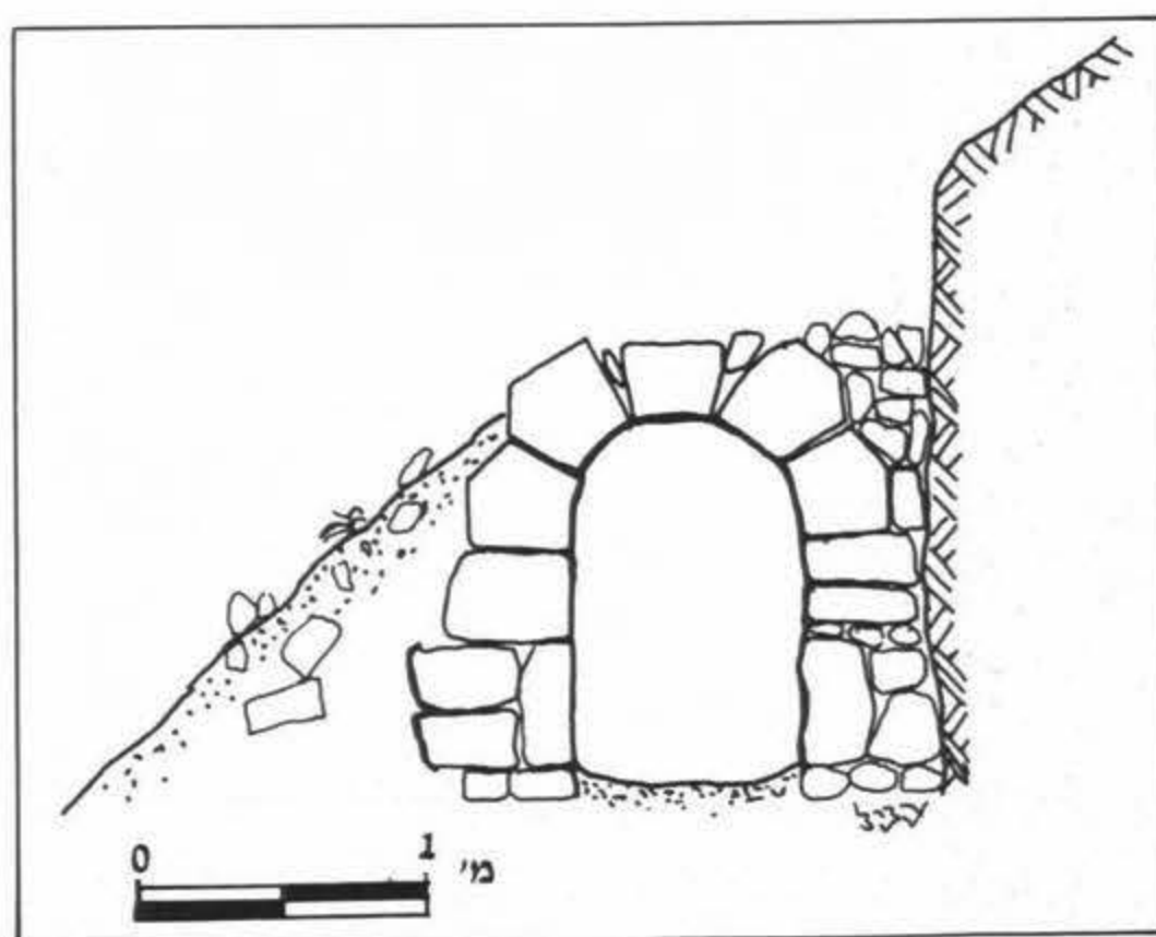
איור 25א: מנהרה מקומרת במדרון הדרומי, חתך
