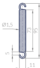
MUELLE RECUPERADOR FALLEBA MRFEX16001
