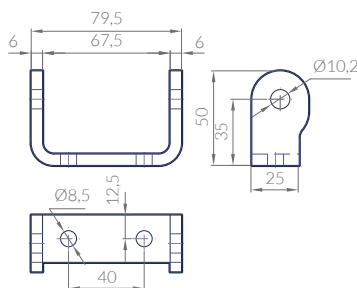
SOPORTE U 25 SBT1MB
