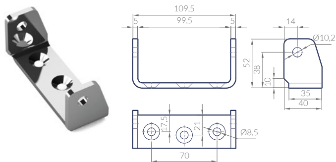
SOPORTE U 40 SBT2B PARA BISAGRA TRASERA HINGE BRACKET U 40 BOCK IN U-FORM 40 CHAPE U 40
