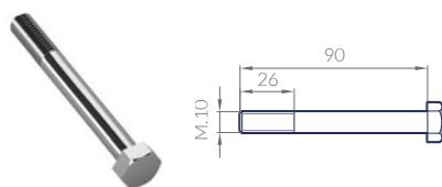
TORNILLO TBT1MA M10X90
