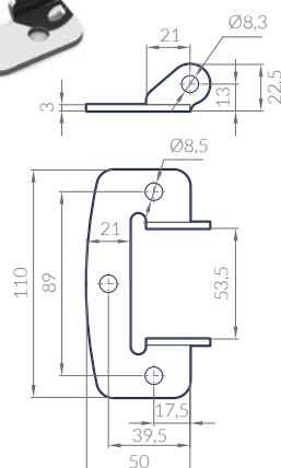
SOPORTE L SBL1MB PARA BISAGRA LATERAL HINGE BRACKET L BOCK IN L-FORM CHAPE L
