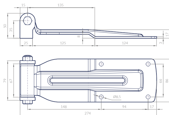
REF-1140201020010202 INOX - S.S. - 862 g
