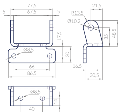
SOPORTE ESCUADRA 30 SBT1MA
