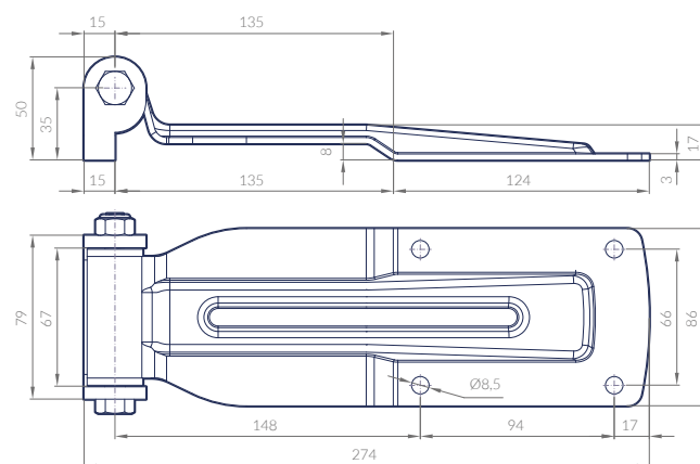
REF-1140201020010203 INOX - S.S. - 826 g
