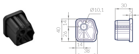
CASQUILLO IZQUIERDO CBT2A PALA BISAGRA TRASERA LEFT BUSH KUNSTSTOFFBUCHSE LINKS DOUILLE
