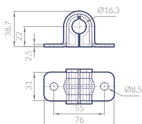
KIT BRIDA CON CASQUILLO 31-16 KB3A KIT TUBE CLAMP WITH BUSH 31-16 KIT ROHRHALTER MIT NYLONBUCHSE 31-16 KIT SUPPORT TUBE AVEC PALIER 31-16
