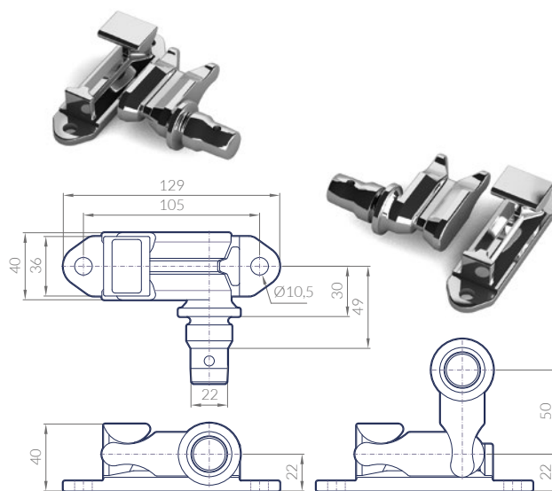
KIT LEVAS- CREMONAS 27 KLC-EX11 PIVOTE CORTO KIT CAMS AND KEEPERS 27 WITH SHORT PIVOT SCHLISSHAKEN UND GEGENHALTER 27 KIT MIT KURZEM SCHAFT KIT PÈNES ET GÂCHES 27 AVEC PIVOT COURT
