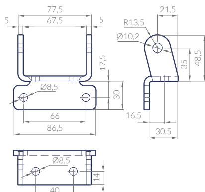
SOPORTE ESCUADRA 30 SBT1MA PARA BISAGRA TRASERA HINGE BRACKET SQUARE BOCK WINKELFORM CHAPE ÉQUÉRRE
