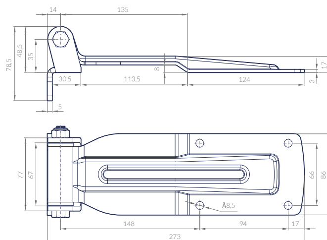
REF-1140201020010201 INOX - S.S. - 937 g
