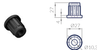
CASQUILLO CBT1MA PALA BISAGRA TRASERA BUSH KUNSTOFFBUCHSE FÜR RÜCKSCHARNIER-BLATT DOUILLE
