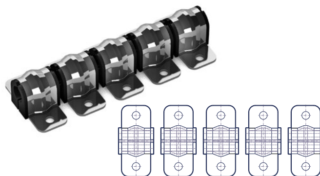
KIT BRIDAS CON CASQUILLO (5X31) - 16 KB3D KIT TUBE CLAMPS WITH BUSH (5X31) - 16 KIT ROHRHÄLTER MIT NYLONBUCHSE (5X31) - 16 KIT SUPPORTS TUBE AVEC PALIER (5X31) - 16
