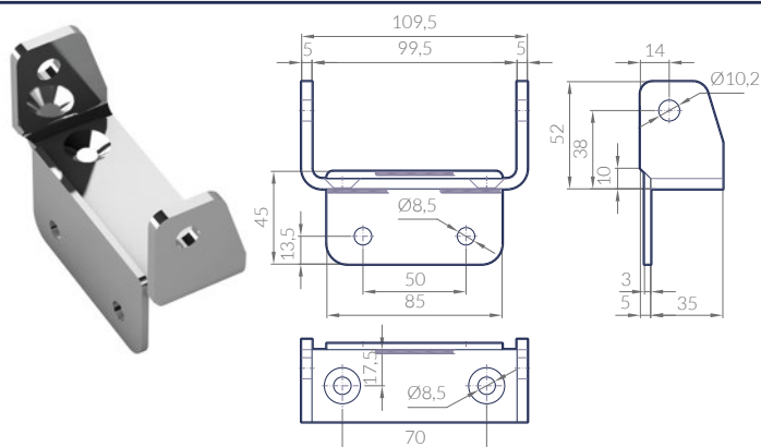
SOPORTE ESCUADRA SBT2A PARA BISAGRA TRASERA HINGE BRACKET SQUARE BOCK WINKELFORM CHAPE ÉQUERRE
