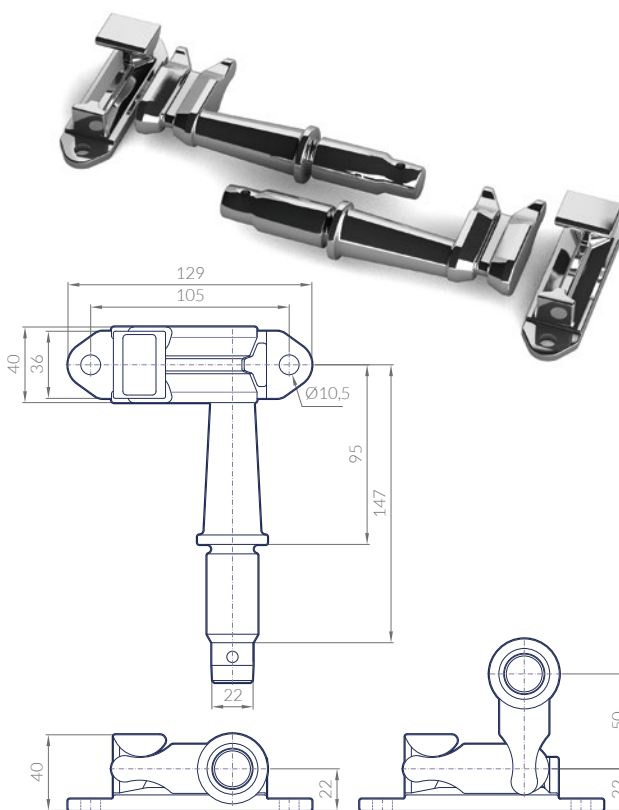
KIT LEVAS-CREMONAS 27 KLC-EX12 PIVOTE LARGO KIT CAMS AND KEEPERS 27 WITH LONG PIVOT SCHLISSHAKEN UND GEGENHALTER 27 KIT MIT LANGEM SCHAFT KIT PÈNES ET GÂCHES 27 AVEC LONG PIVOT
