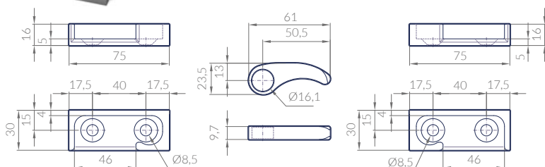
KIT DE LEVAS - CREMONAS EMPOTRAR KLC-EM2 KIT RECESSED CAMS+ KEEPERS KIT EINBAUSCHLISSKEILE U. GEGENHALTER KIT PÈNES ET GÂCHES À ENCASTER
