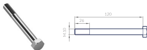
TORNILLO M10X120 DIN 931 TBT2A PIN BOLZEN AXE
