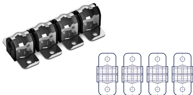
KIT BRIDAS CON CASQUILLO (4X31) - 16 KB3C KIT TUBE CLAMPS WITH BUSH (4X31) - 16 KIT ROHRHÄLTER MIT NYLONBUCHSE (4X31) - 16 KIT SUPPORTS TUBE AVEC PALIER (4X31) - 16
