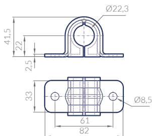
KIT BRIDA CON CASQUILLO 33-22 KB2A KIT TUBE CLAMP WITH BUSH 32-22 KIT ROHRHALTER MIT NYLONBUCHSE 32-22 KIT SUPPORT TUBE AVEC PALIER 32-22 KB2A REF-1120100020010202 INOX - S.S. - 91 g
