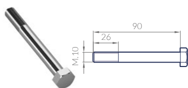
TORNILLO TBT1MA M10X90 DIN 931 PIN | BOLZEN | AXE
