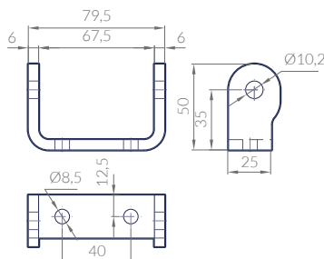
SOPORTE U 25 SBT1MB PARA BISAGRA TRASERA HINGE BRACKET U 25 BOCK IN U-FORM 25 CHAPE U 25
