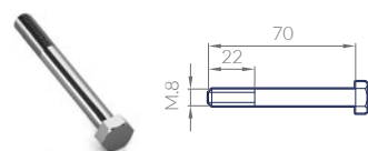
TORNILLO M8X70 DIN 931 TBL1MA PIN | BOLZEN | AXE
