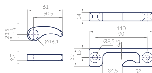
KIT DE LEVAS - CREMONAS EMPOTRAR KLC-EM1 KIT RECESSED CAMS+KEEPERS KIT EINBAUSCHLISSKEIL U. GEGENHALTER KIT PÈNES ET GÂCHES À ENCASTER
