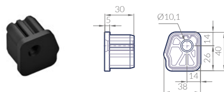
CASQUILLO DERECHO CBT2A PALA BISAGRA TRASERA RIGHT BUSH KUNSTSTOFFBUCHSE RECHTS DOUILLE
