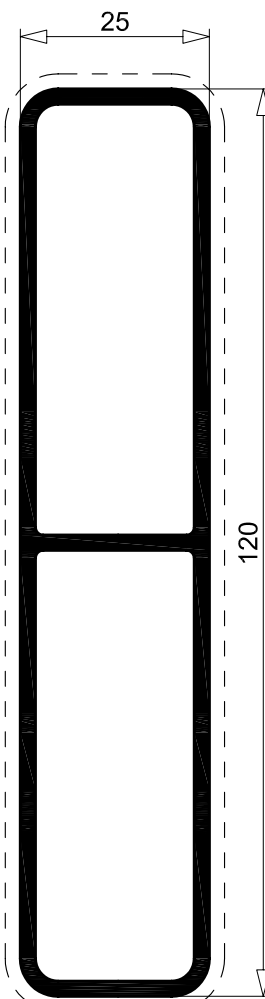
R 1266 1.603 Kg/m sup. in vista 281 mm per. esterno 281 mm
