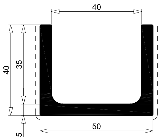
B 1142 1.647 Kg/m sup. in vista 129 mm per. esterno 244 mm
