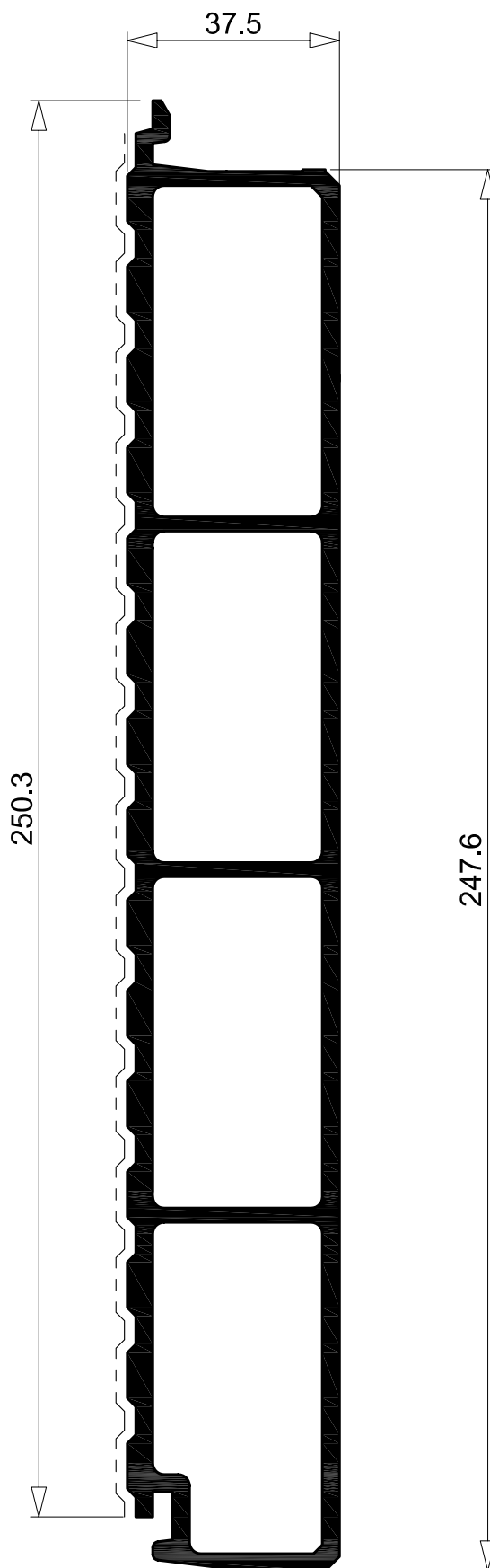
R 4319 5.854 Kg/m sup. in vista 263 mm per. esterno 623 mm
