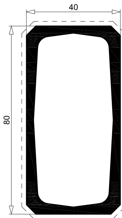
MR 793 2.219 Kg/m sup. in vista 230 mm per. esterno 230 mm
