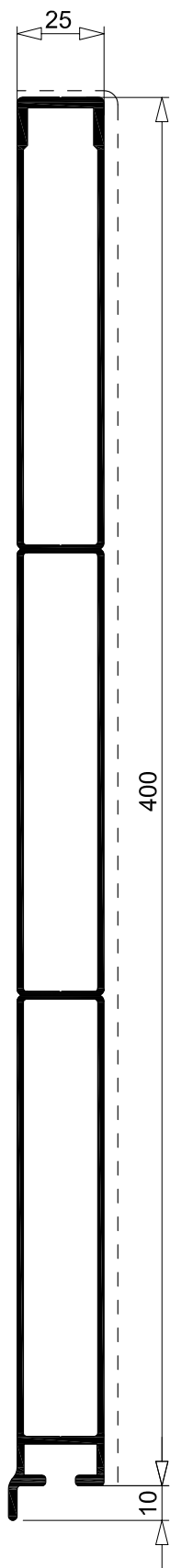
R 4505 4.700 Kg/m sup. in vista 400 mm per. esterno 920 mm
