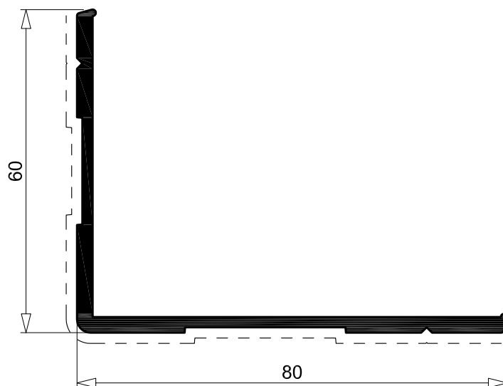
AI 0026 0.926 Kg/m sup. in vista 142 mm per. esterno 284 mm
