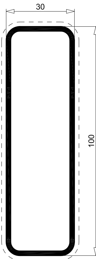
R 1198 1.300 Kg/m sup. in vista 260 mm per. esterno 260 mm
