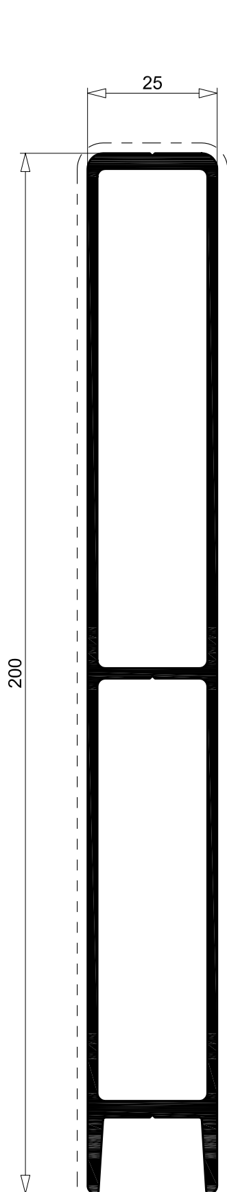
R 3406 2.565 Kg/m sup. in vista 425 mm per. esterno 475 mm
