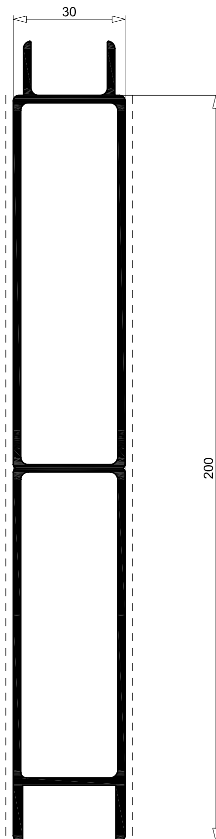
R 3407 2.754 Kg/m sup. in vista 400 mm per. esterno 550 mm
