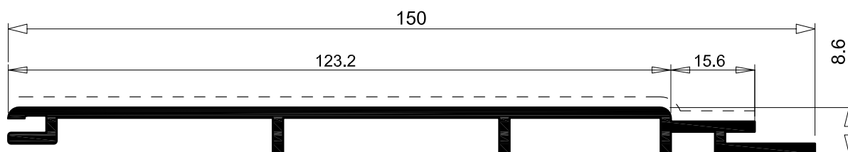
I 3496 0.976 Kg/m sup. in vista 139 mm per. esterno 385 mm
