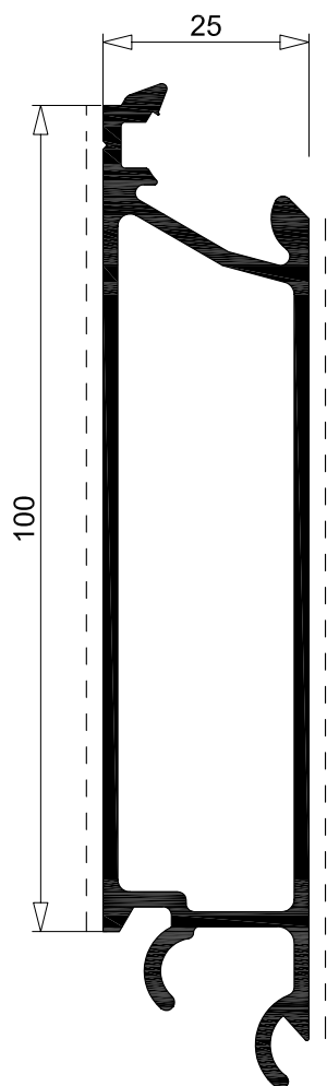
R 7350 1.482 Kg/m sup. in vista 198 mm per. esterno 353 mm
