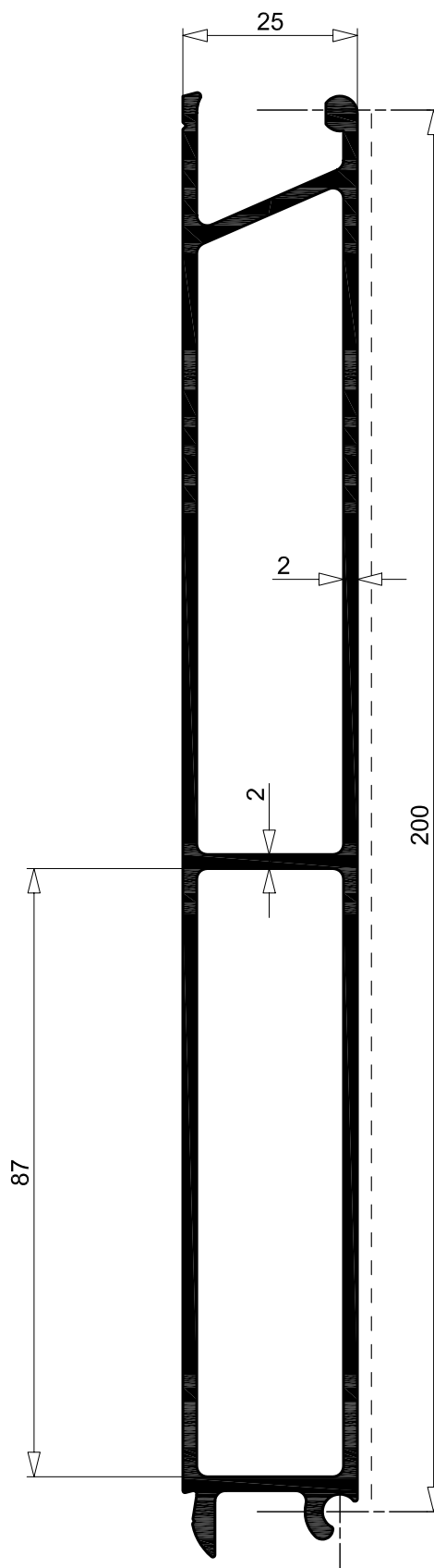
R 1632 2.500 Kg/m sup. in vista 200 mm per. esterno 524 mm
