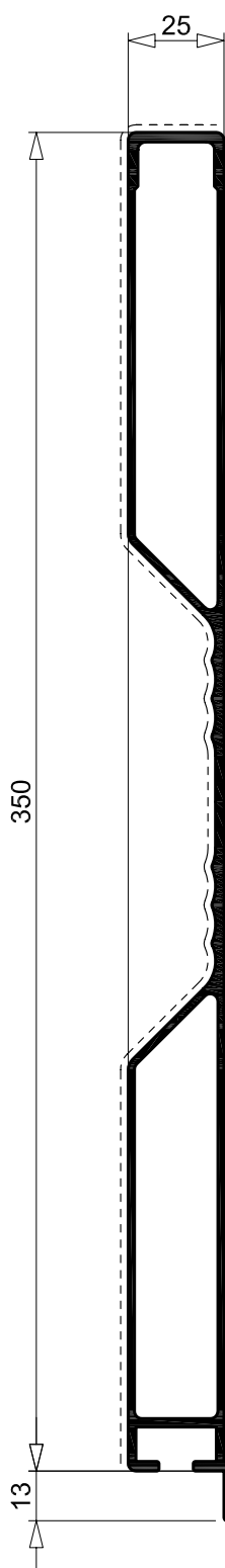
R 7029 3.453 Kg/m sup. in vista 390 mm per. esterno 841 mm
