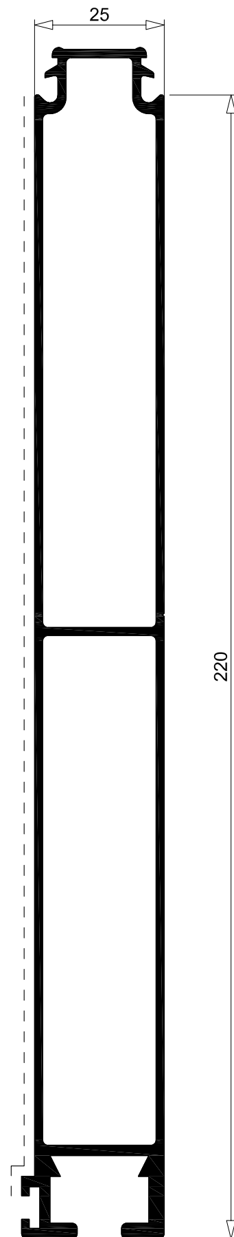
R 3475 2.581 Kg/m sup. in vista 120 mm per. esterno 397 mm
