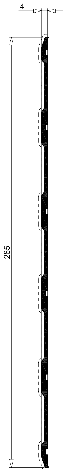
I 6794 2.184 Kg/m sup. in vista 296 mm per. esterno 600 mm
