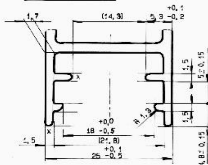
DETAIL M2:1
