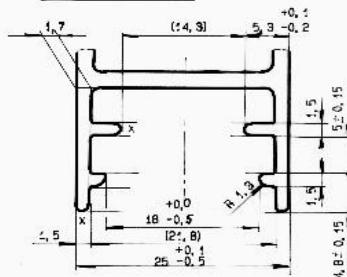
DETAIL M2:1
