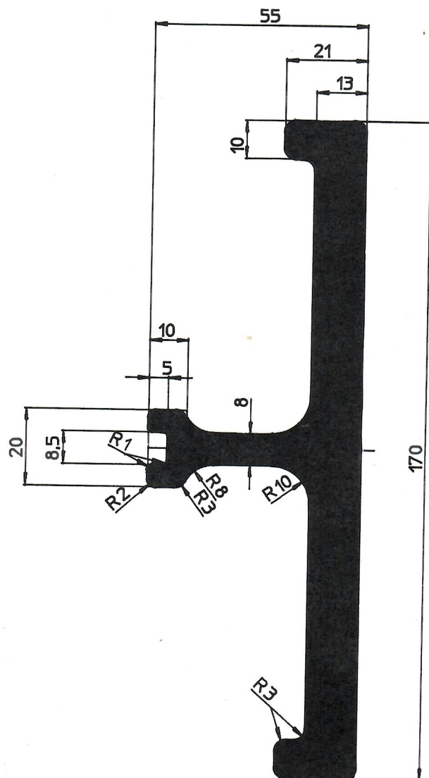
7528 Profil zákl. rámu
