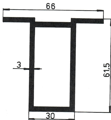
4929 (B) příčný nosník
