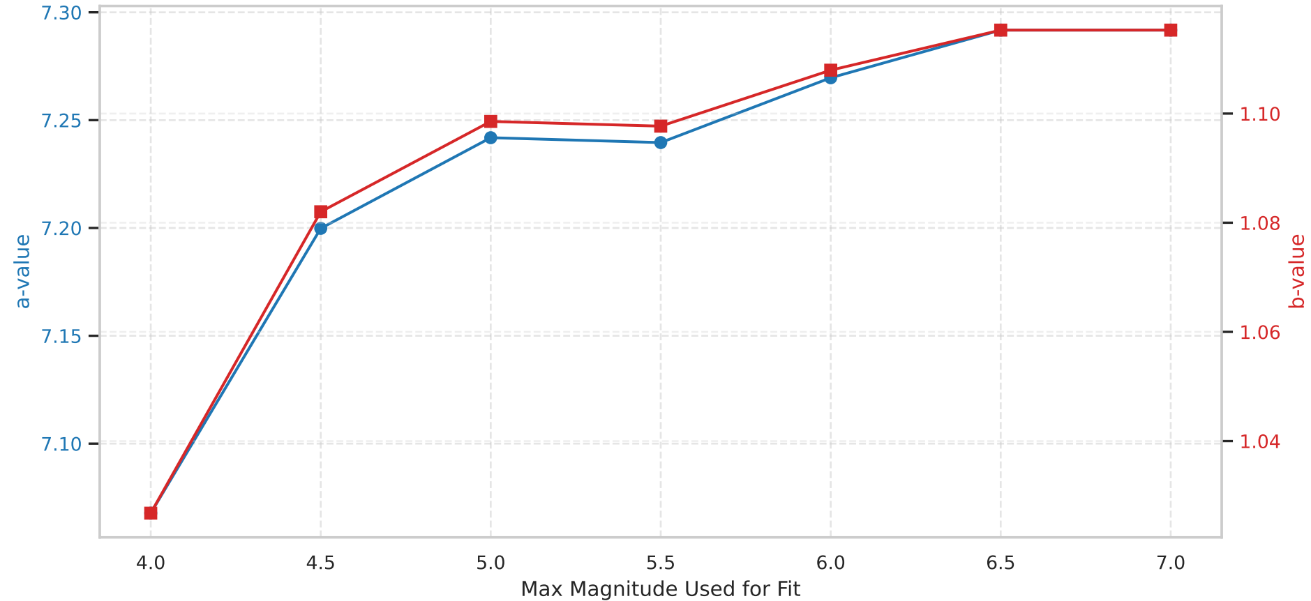
Gutenberg-Richter Parameters vs Max Magnitude
