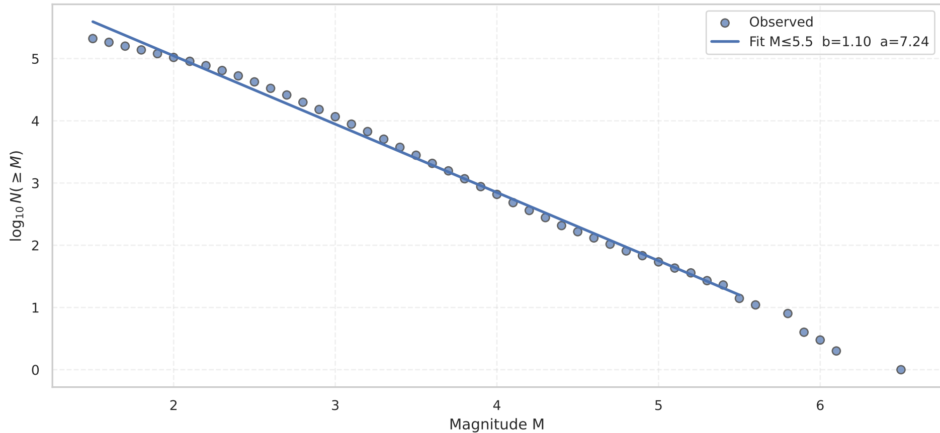
Gutenberg-Richter ( M \leq 5.5 )
