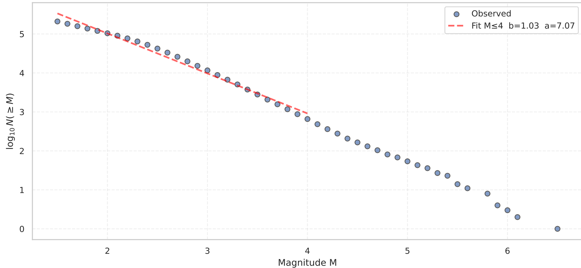
Gutenberg-Richter ( M \leq 4 )
