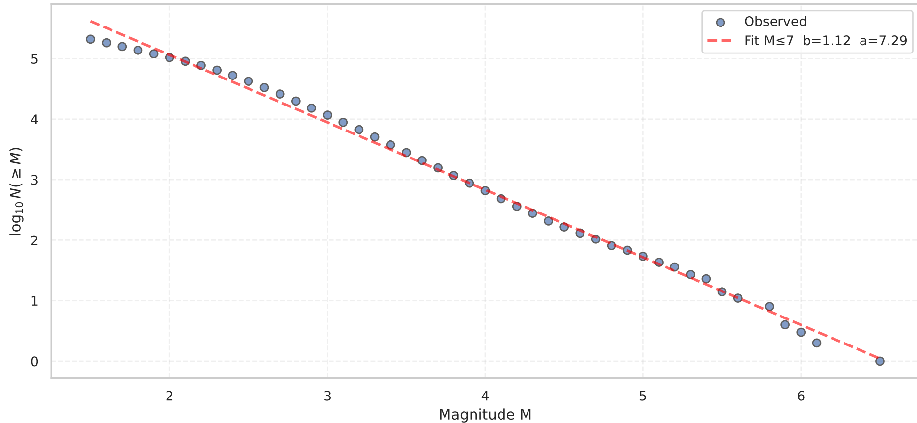
Gutenberg-Richter ( M \leq 7 )
