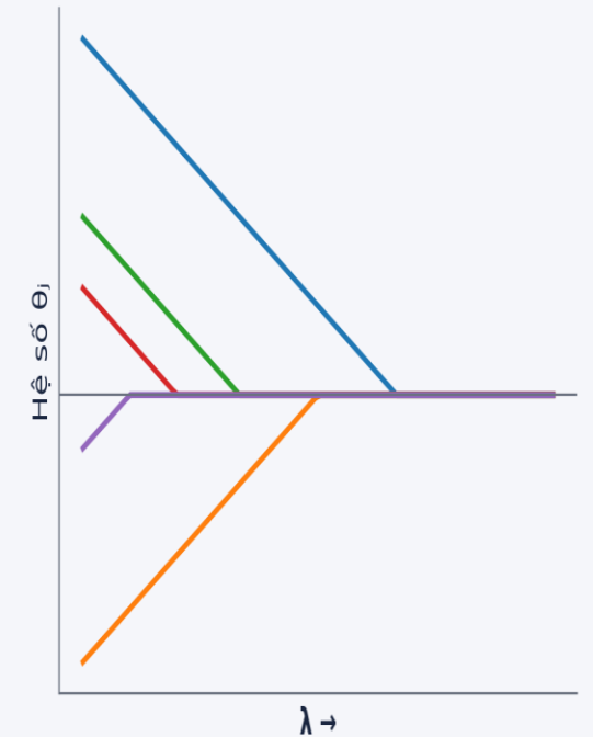
Lasso (L1): nhiều hệ số về ĐÚNG 0
