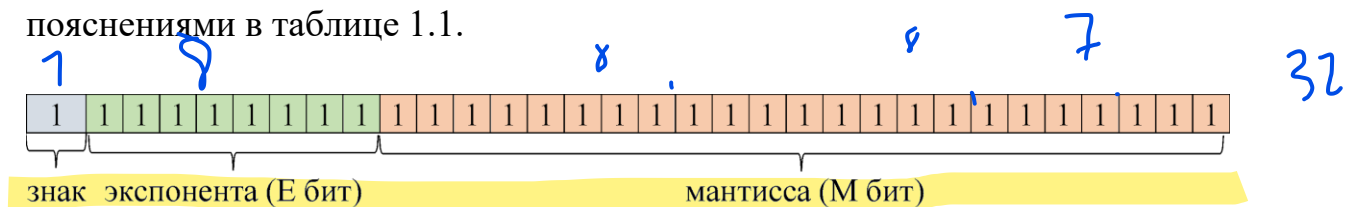
Рисунок 1.1 – Битовое представление вещественного числа
