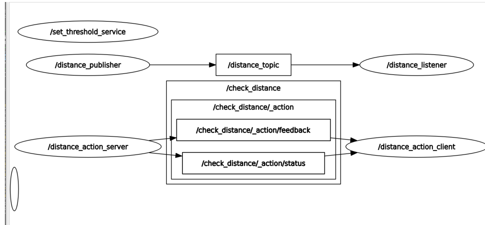
rqt_graph
