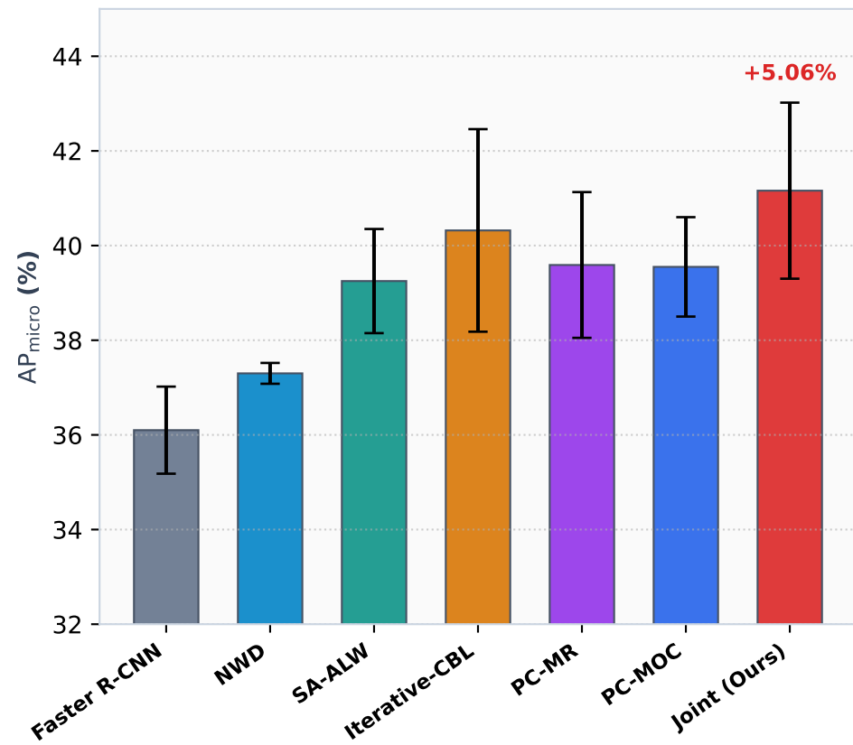
(a) AP micro (Sub-8 × 8 px)
