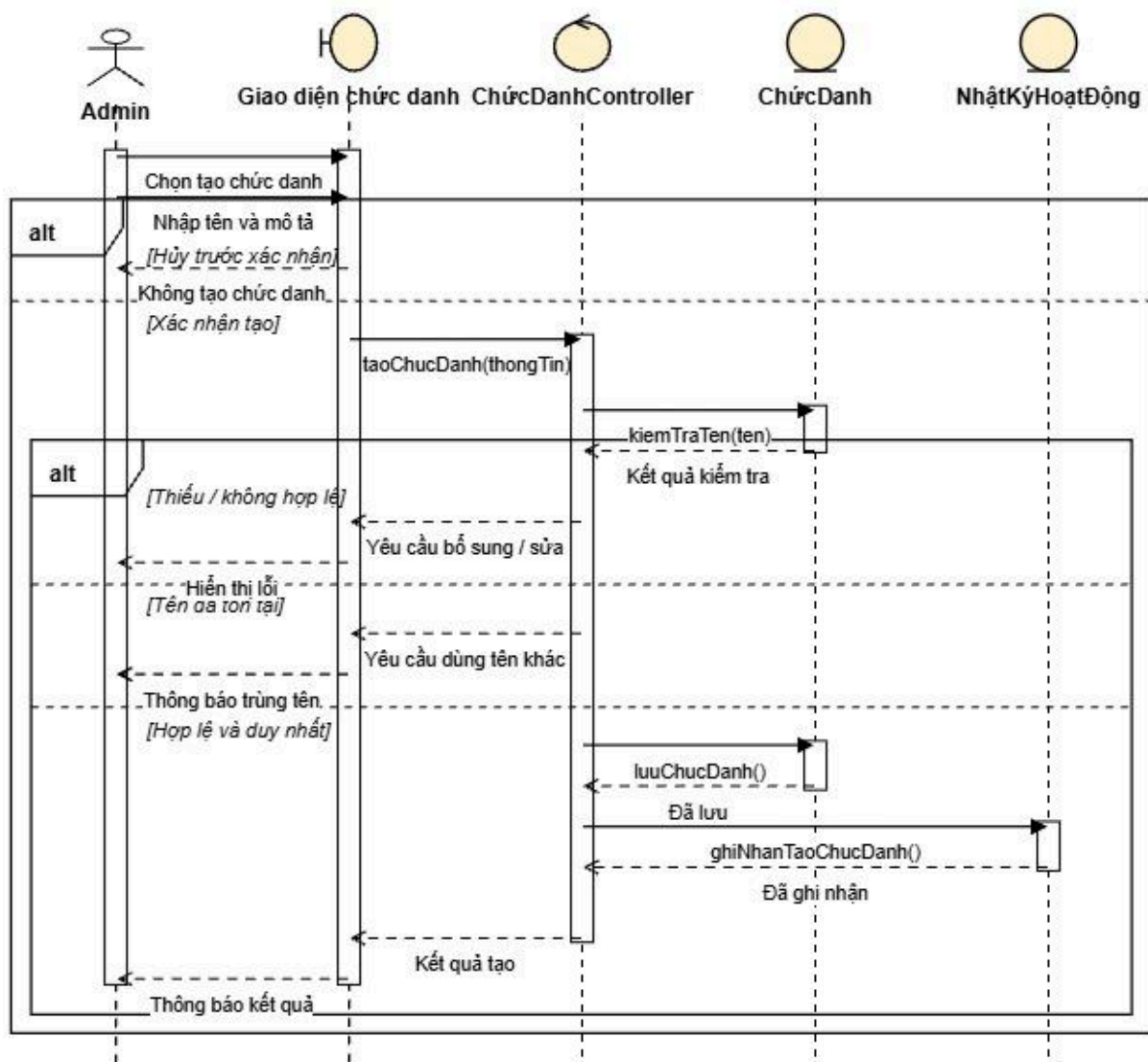
Hình 2.40. Biểu đồ tuần tự - Tạo chức danh
