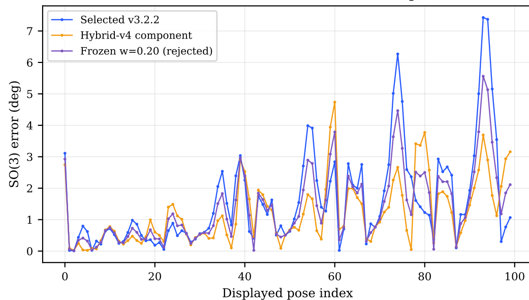
(d) Orientation error — no smoothing
