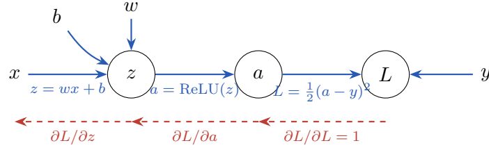
Hình 2: Computational graph của z = wx + b \rightarrow a = \text{ReLU}(z) \rightarrow L = \frac{1}{2}(a - y)^2 . Mũi tên xanh (liền) = forward; mũi tên đỏ (đứt) = backward, đi ngược đúng theo các cạnh forward.
