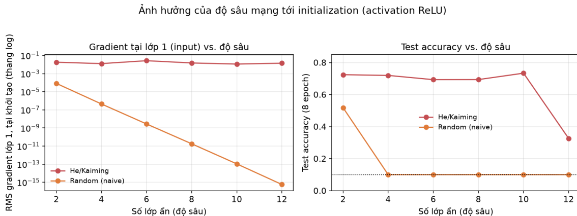
Hình 5: Gradient RMS lớp 1 tại khởi tạo (trái) và test accuracy sau 8 epoch (phải), theo độ sâu mạng, activation ReLU. Đường chấm ở đồ thị phải = mức ngẫu nhiên (10%).
