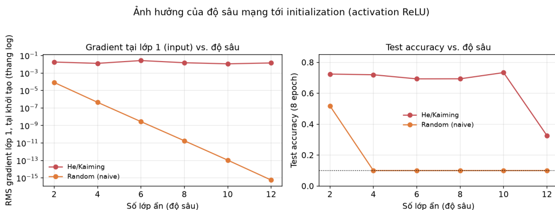
Hình 5: Gradient RMS lớp 1 tại khởi tạo (trái) và test accuracy sau 8 epoch (phải), theo độ sâu mạng, activation ReLU. Đường chấm ở đồ thị phải = mức ngẫu nhiên (10%).
