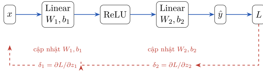
Hình 3: Gradient đi ngược Loss \rightarrow Output \rightarrow Hidden \rightarrow Input. Mỗi \delta_l = \partial L/\partial z_l được tính một lần rồi dùng lại cho mọi tham số của lớp l — đây là điểm làm Backprop hiệu quả (Mục 4.4).
