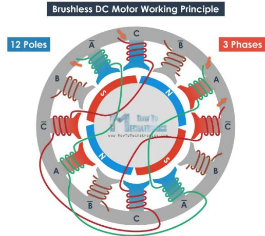
b) Poles in a BLDC motor
