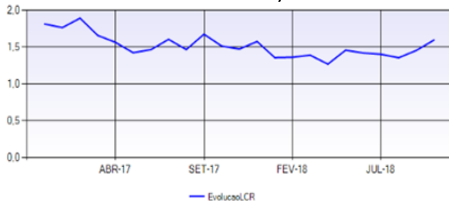
LCR - Proxy
