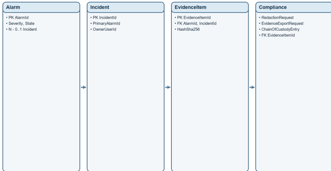
Hình 4.15. ERD chi tiết SOC & Evidence
