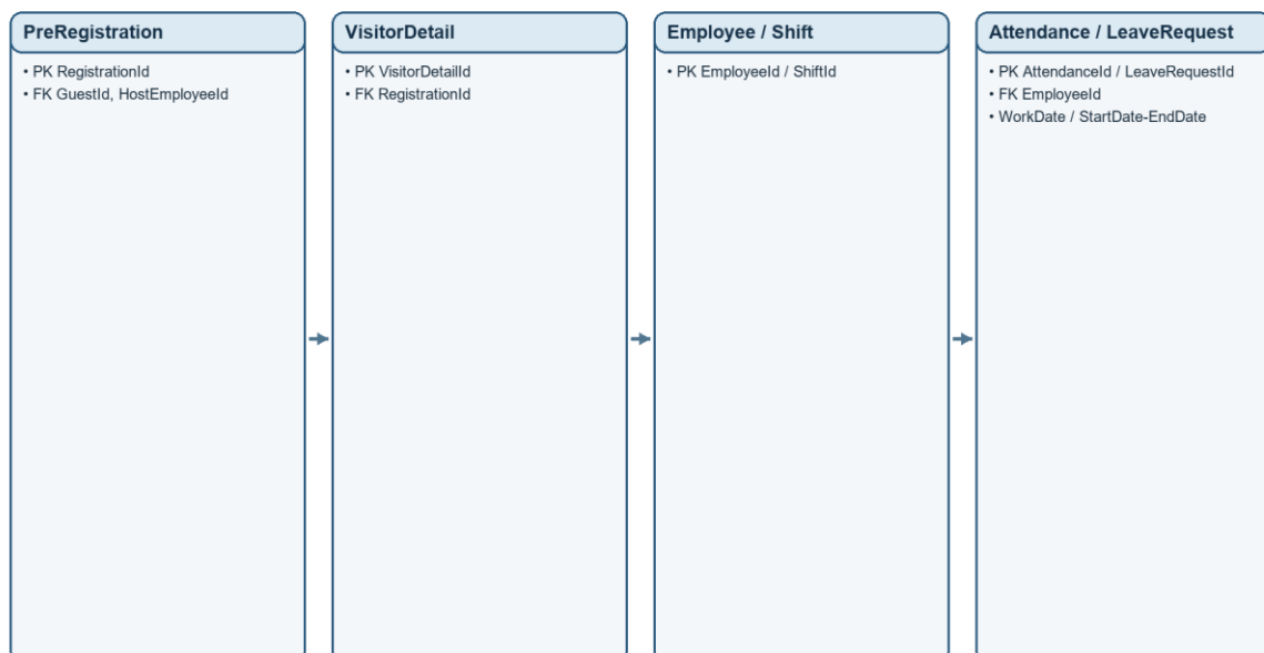
Hình 4.14. ERD chi tiết Visitor & HR
