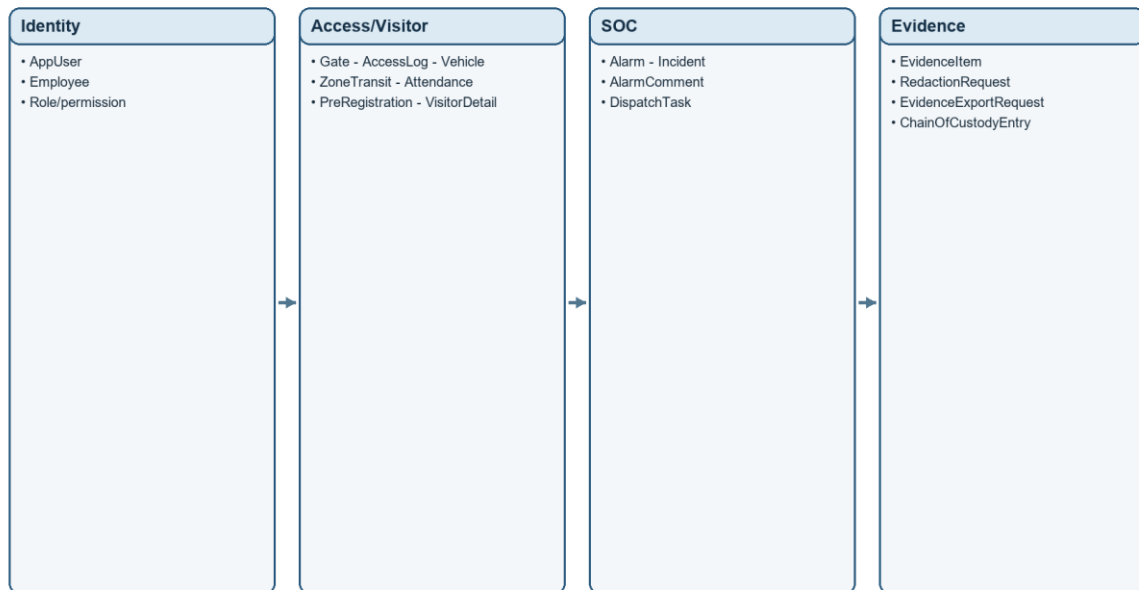
Hình 4.12. ERD tổng quan V-Shield 2.0
