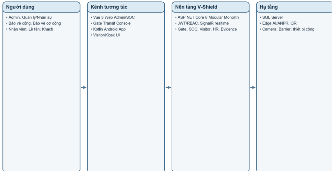
Hình 3.1. Mô hình tổng quan hệ thống V-Shield 2.0
