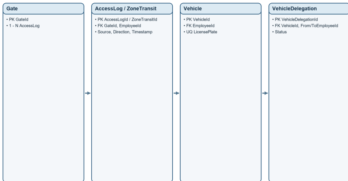
Hình 4.13. ERD chi tiết Access & Vehicle
