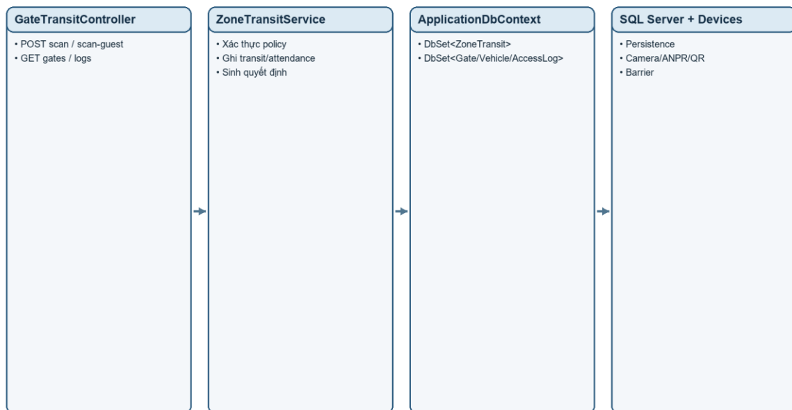
Hình 4.16. Class / Repository Diagram module Gate Transit
