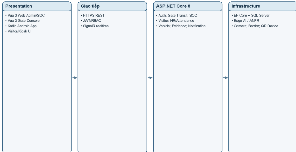
Hình 4.1. Kiến trúc công nghệ V-Shield 2.0
