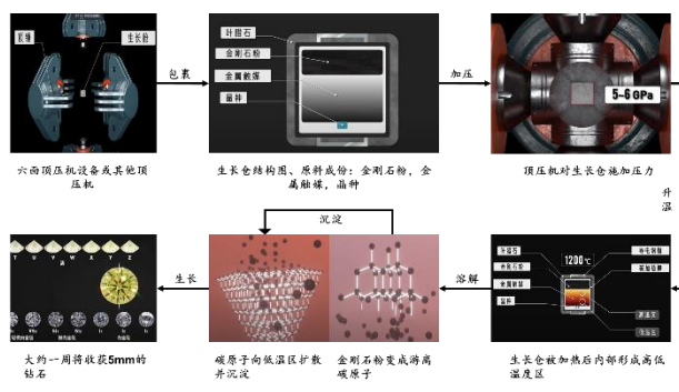
图表25： 高温高压法流程
