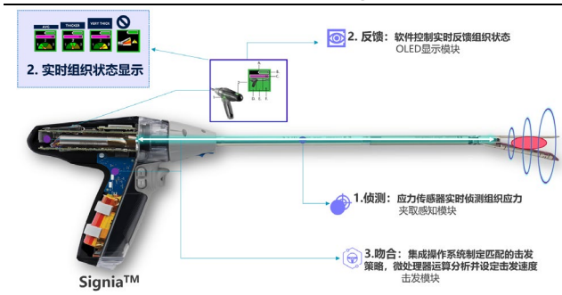
图表 32.美敦力智能吻合平台 Signia
