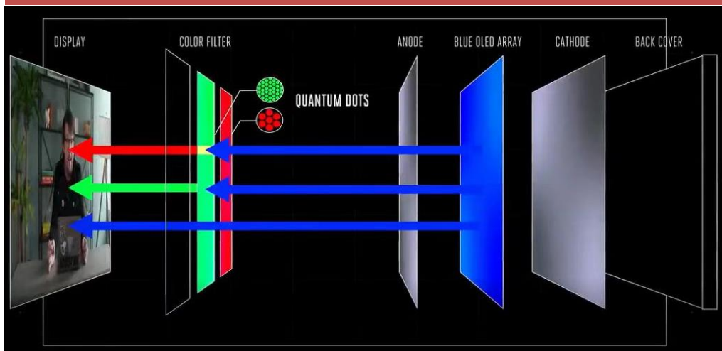
QD-OLED电视结构
