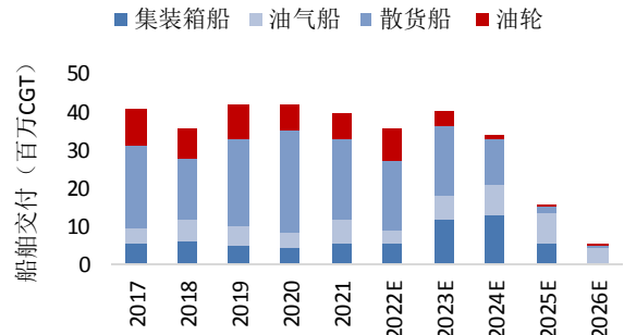
图 6：根据船舶计划交付量，2023-24 年船台基本排满
