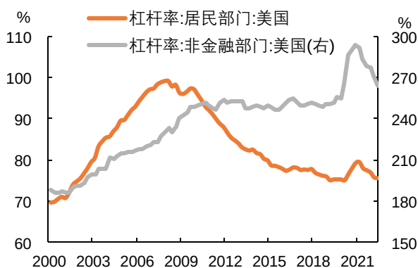
图表21 美国居民杠杆率处于次贷危机以来的低位水平
