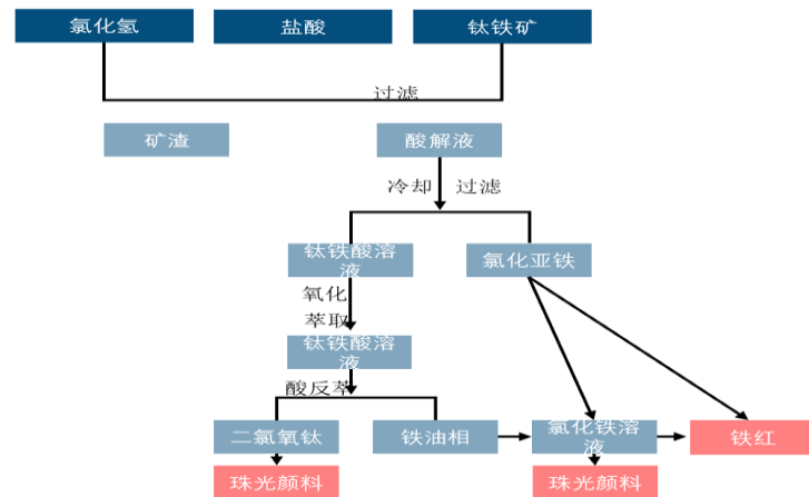
图表：氯化钛萃取分离简化流程
