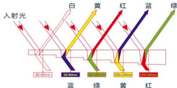
图表：不同金属氧化物厚度决定干涉颜色
