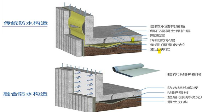
图表：公司融合防水示意图
