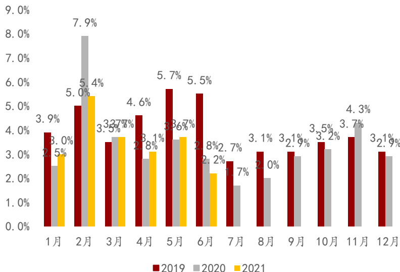
图表15: 2019-2021年全国月度平均弃风率 (%)
