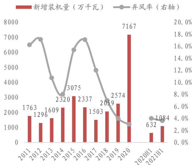
图表14: 2011年-2021H1我国风电新增装机及弃风率
